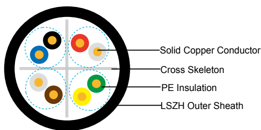
U/UTP CAT6
