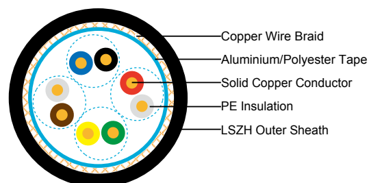
SF/UTP CAT5E
