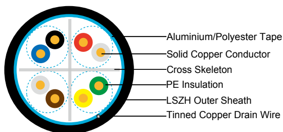
F/UTP CAT6
