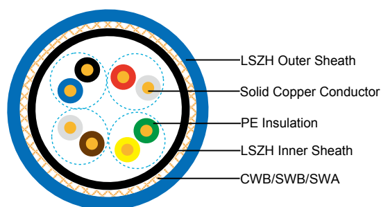
U/UTP CAT5E
